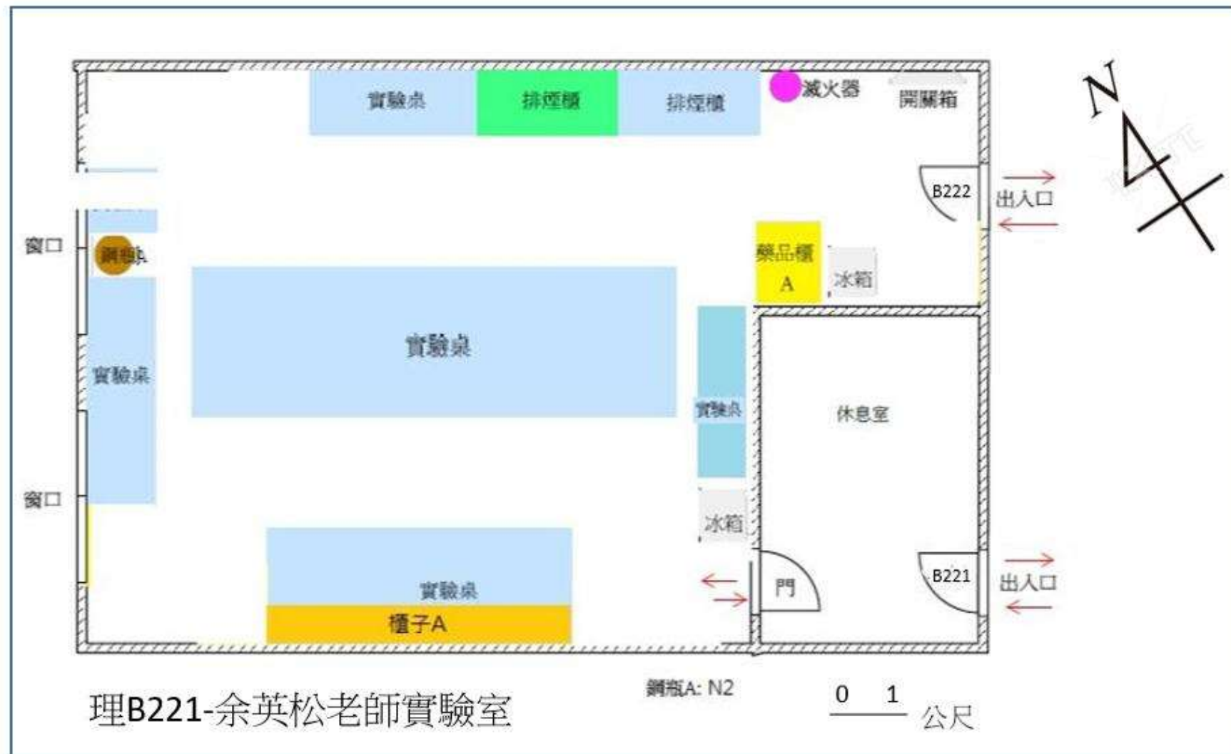
圖二-1、工作場所配置圖
