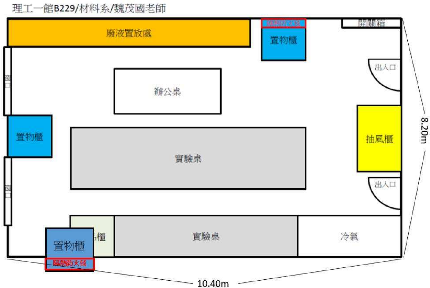
圖二-2、工作場所配置圖
